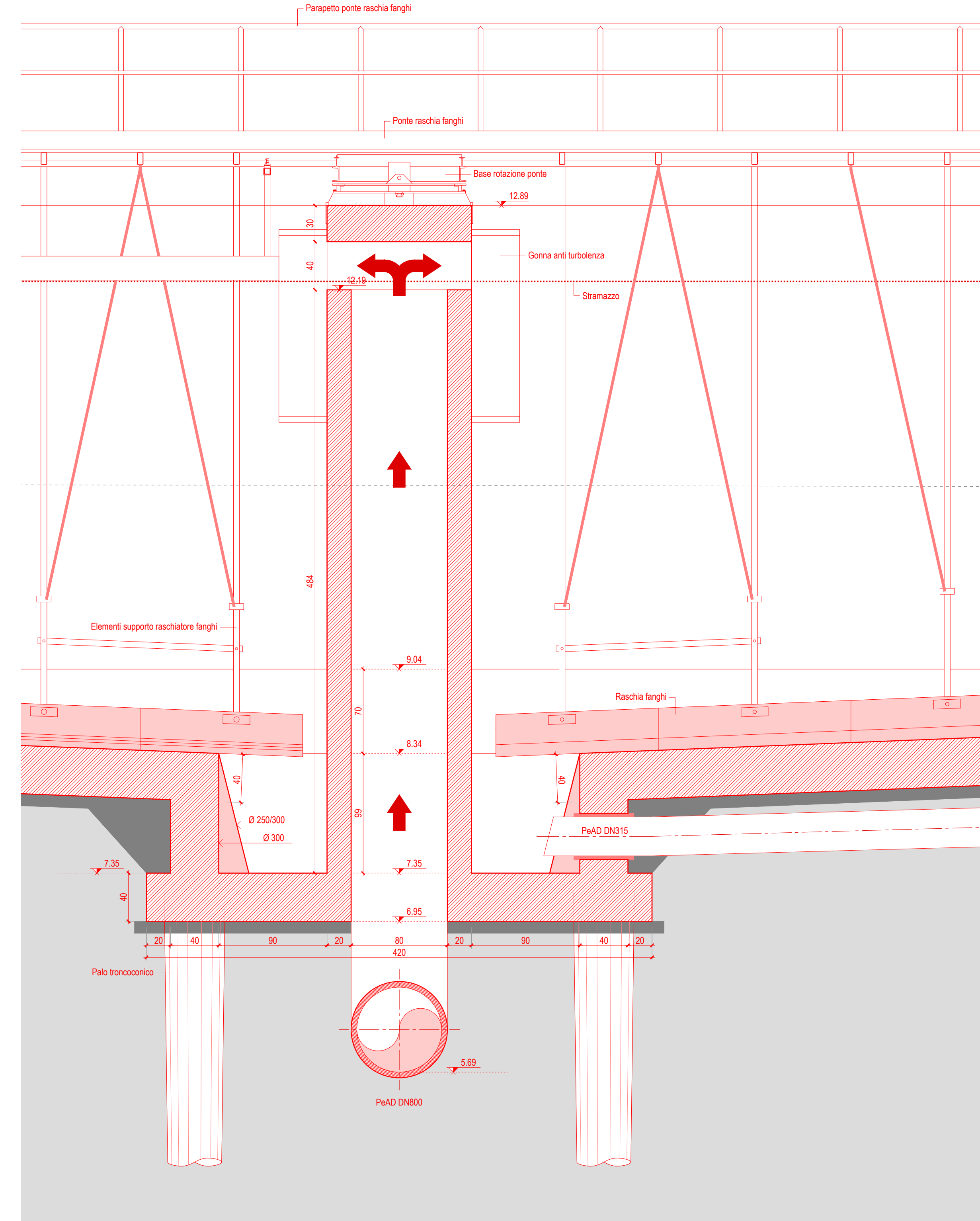
SEDIMENTATORE CIRCOLARE 1 Sezione A-A: VASCA POMPE scala 1:25
