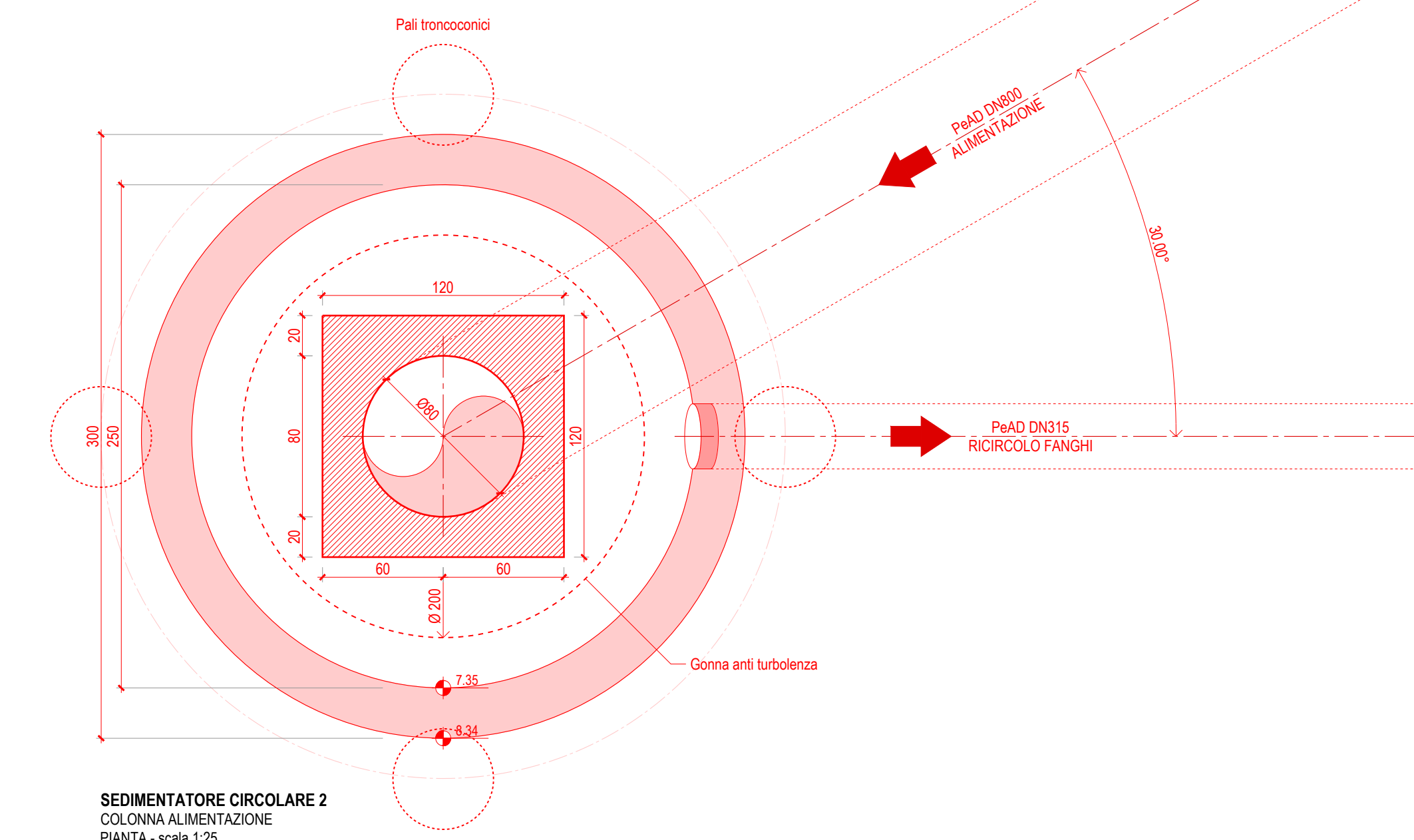
SEDIMENTATORE CIRCOLARE 2 COLONNA ALIMENTAZIONE PANTA - scala 1:25
