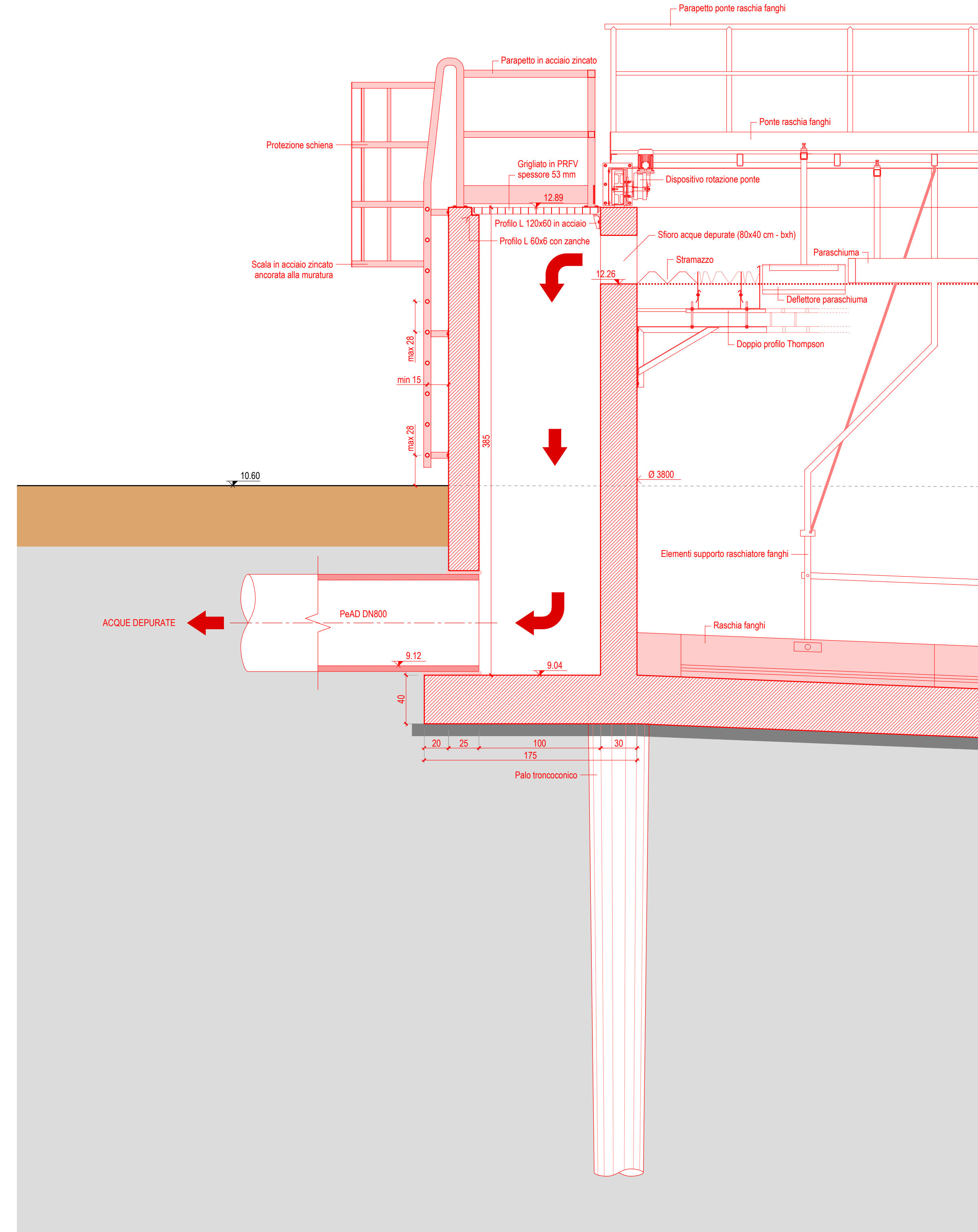
SEDIMENTATORE CIRCOLARE 2 Sezione A-A: COLONNA ALIMENTAZIONE scala 1:25
