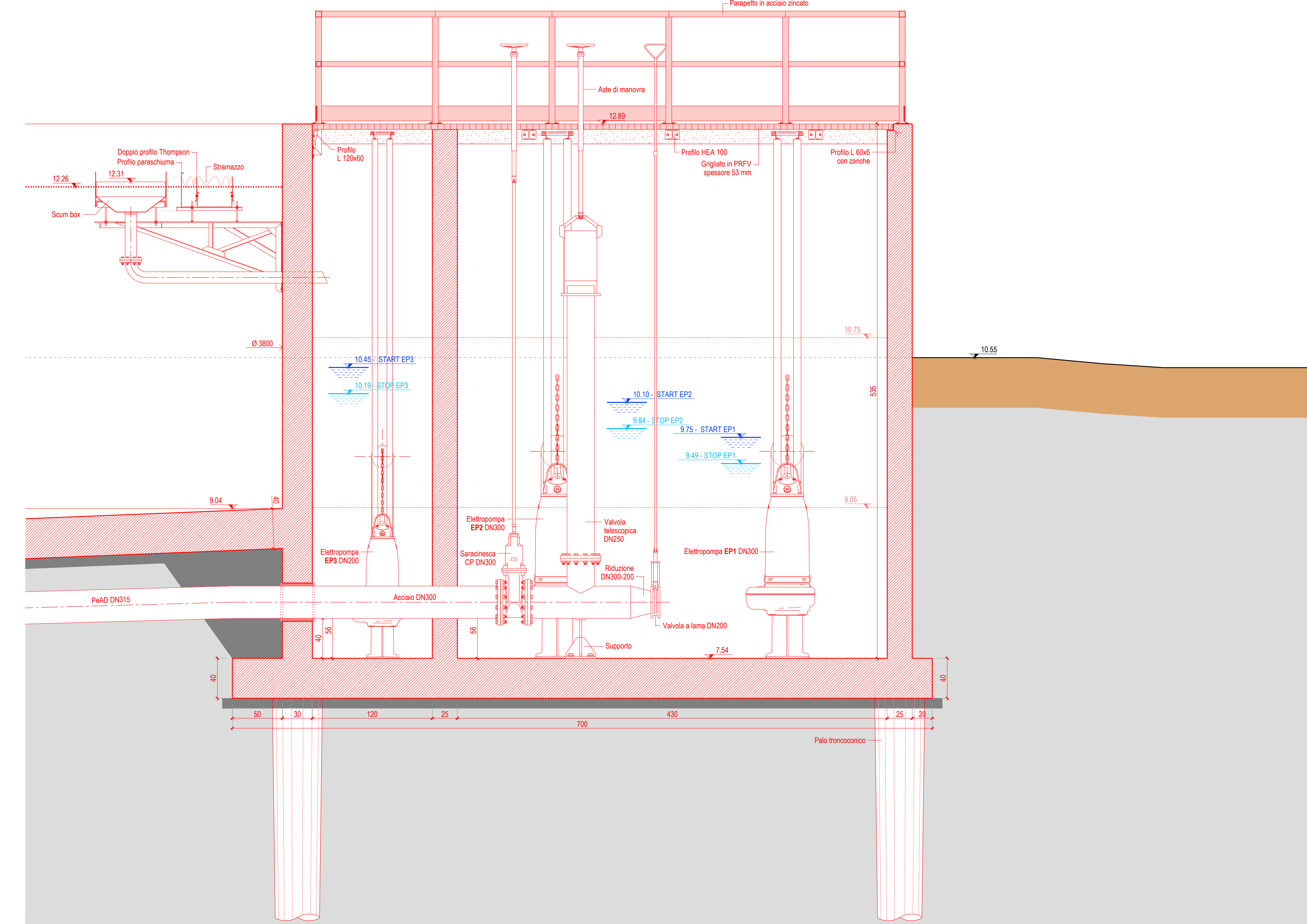
SEDIMENTATORE CIRCOLARE 2 Sezione A-A: VASCA POMPE scala 1:25
