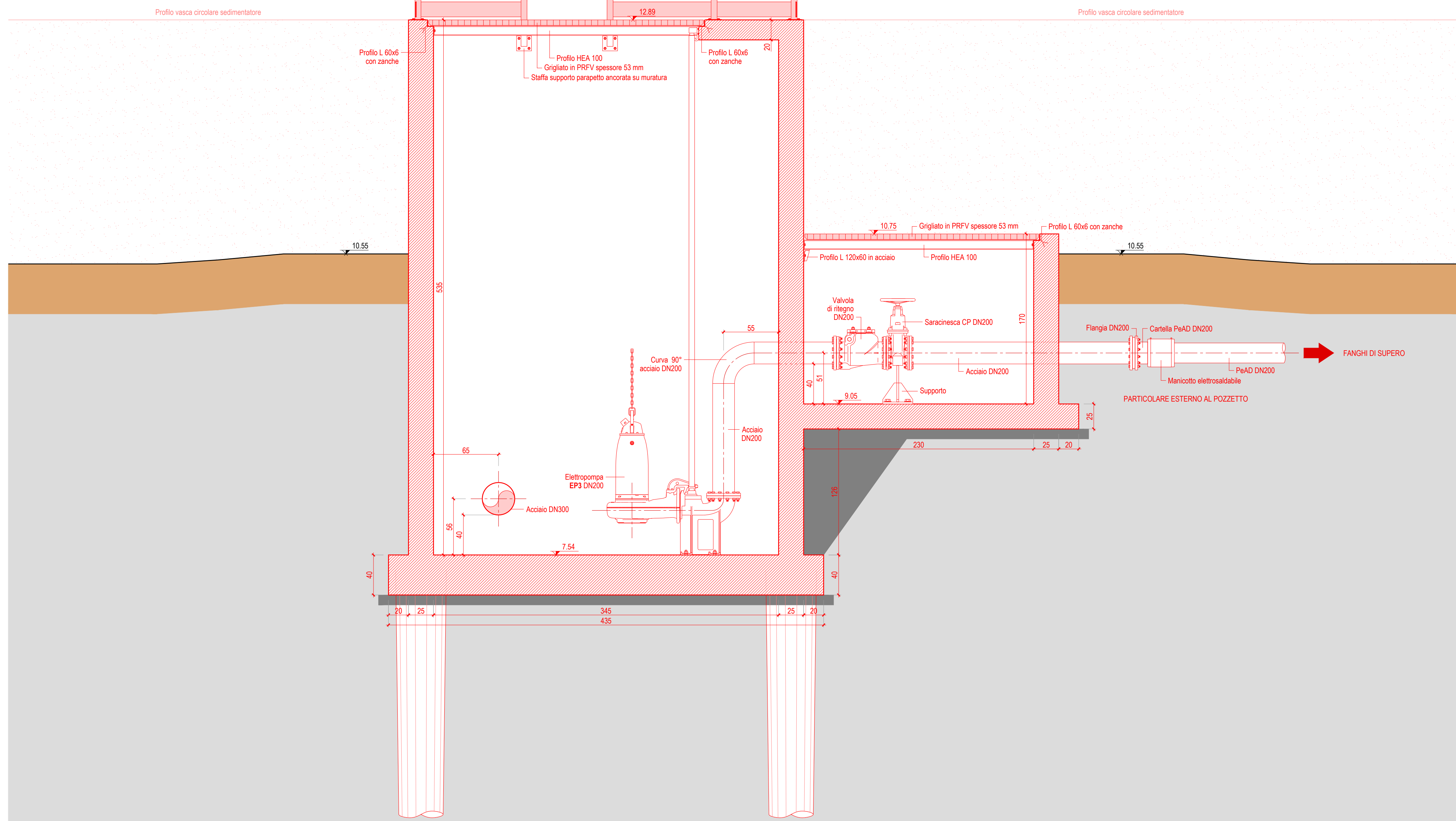
SEDIMENTATORE CIRCOLARE 1 Sezione C-C: VASCA POMPE e CAMERA DI MANOVRA scala 1:25
