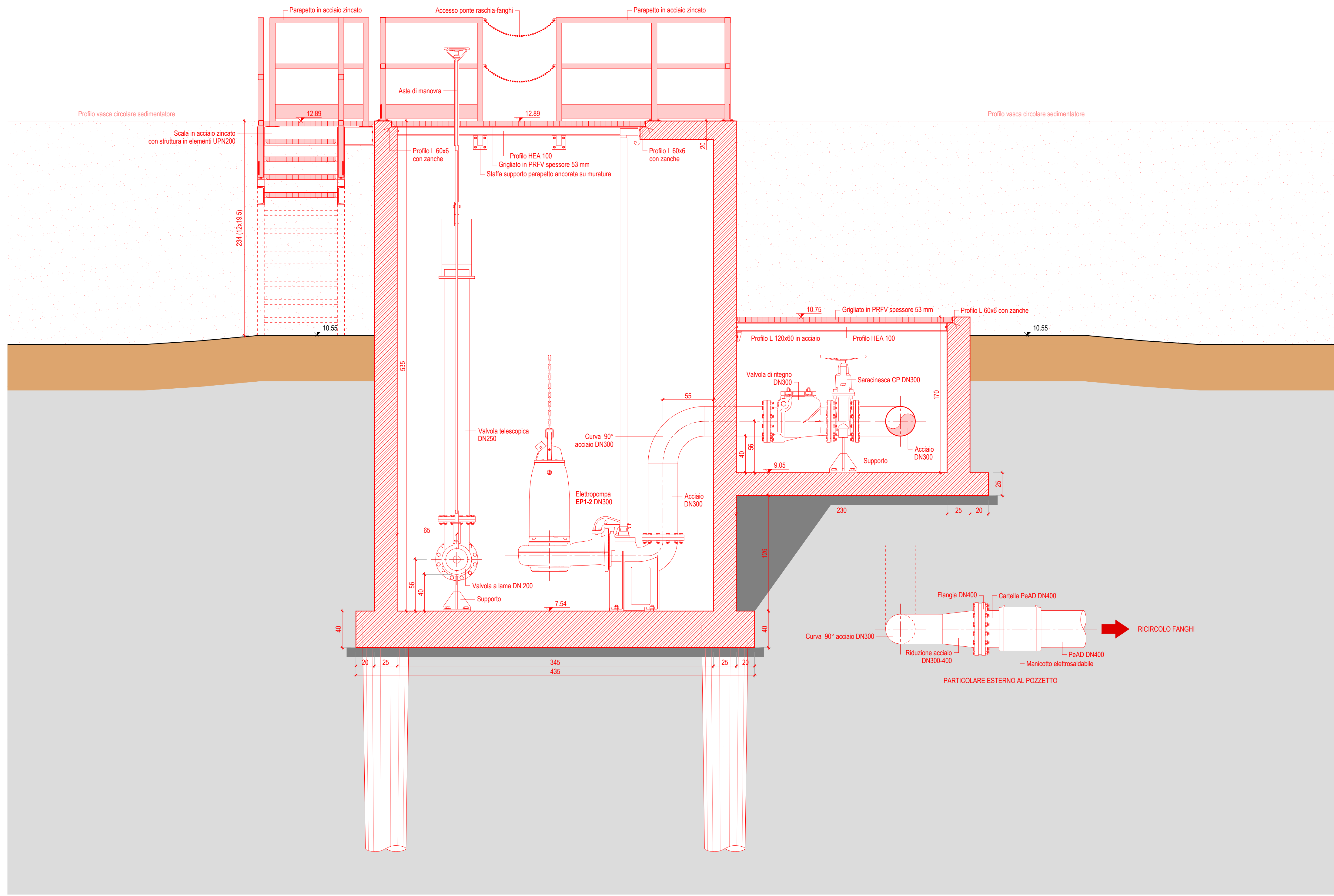
SEDIMENTATORE CIRCOLARE 1 Sezione B-B: VASCA POMPE e CAMERA DI MANOVRA scala 1:25
